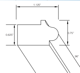
Bottom Edge Molding - BEM8
